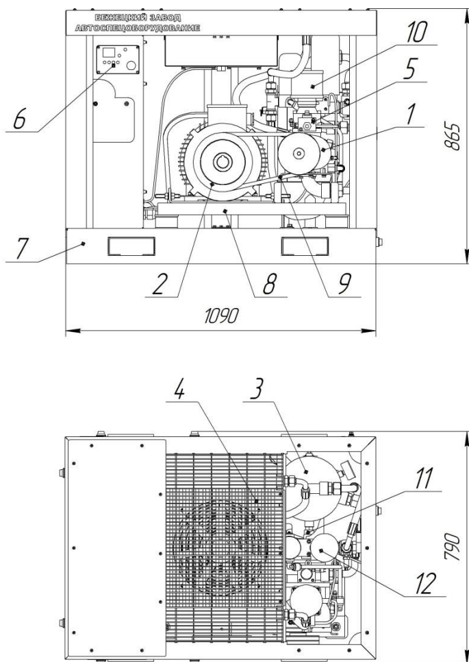
Рисунок 2. Агрегат компрессорный
